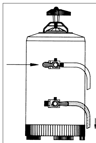
Рис.3 Регенерация
